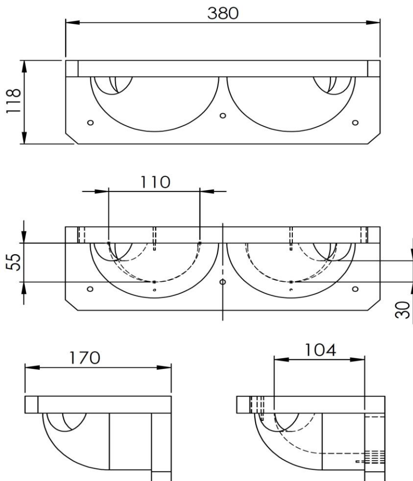
slika 2: dimenzije StoElement Fauna SW-F 20
